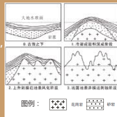
花岗岩地貌形成示意图
